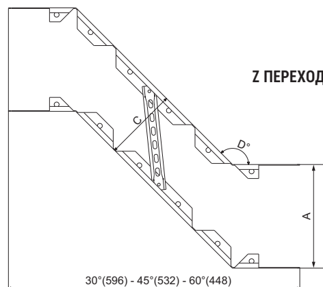
СИММЕТРИЧНЫЙ ПЕРЕХОДНИК
